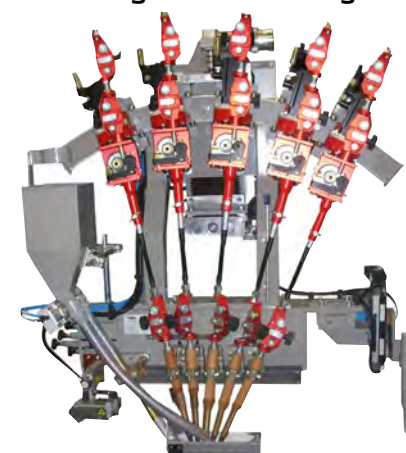
Longitudinal welding
